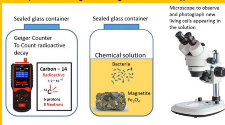
Esemplificazione dell'esperimento con contenitori sigillati, contenenti Carbonio-14 e l'altro soluzione di molecole fondamentali
